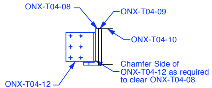
Section A-A ONX-T04-12 and ONX-T04-08 Assembly
